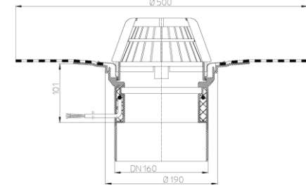
Рис. 4. Кровельная воронка HL62.1H/5.
