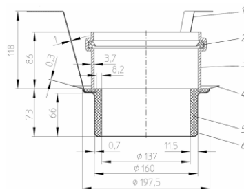
Рис. 7. Противопожарная муфта HL870 для кровельной воронки HL62.1H/1.
