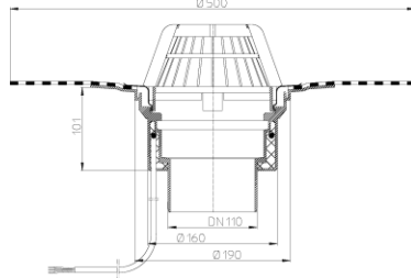
Рис. 2. Кровельная воронка HL62.1H/1.
