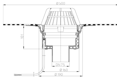
Рис. 1. Кровельная воронка HL62.1H/7.
