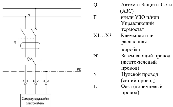
Рис. 5. Схема подключения электрообогрева кровельной воронки HL62.1H к электрической сети.
