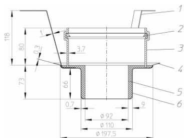
Рис. 6. Противопожарная муфта HL850 для кровельной воронки HL62.1H/7
