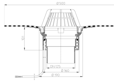
Рис. 3. Кровельная воронка HL62.1H/2.
